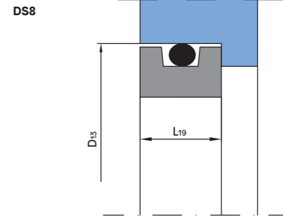
Dimension table Ø 65 – 100 mm
